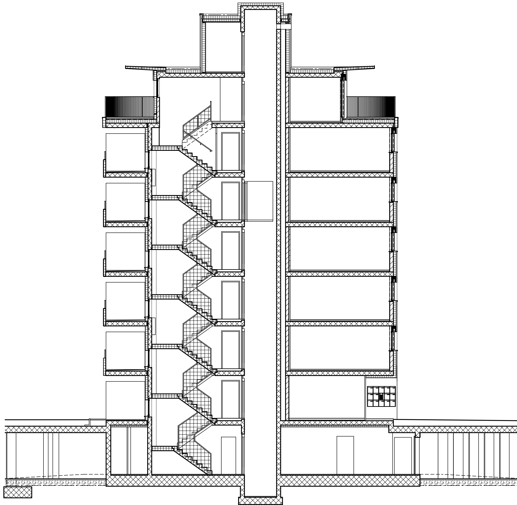
HAUS 5 SCHNITT 1:100
