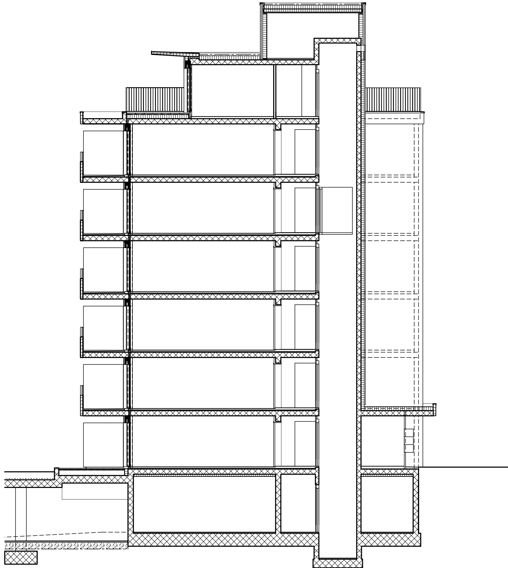
HAUS 2 SCHNITT 1:100
