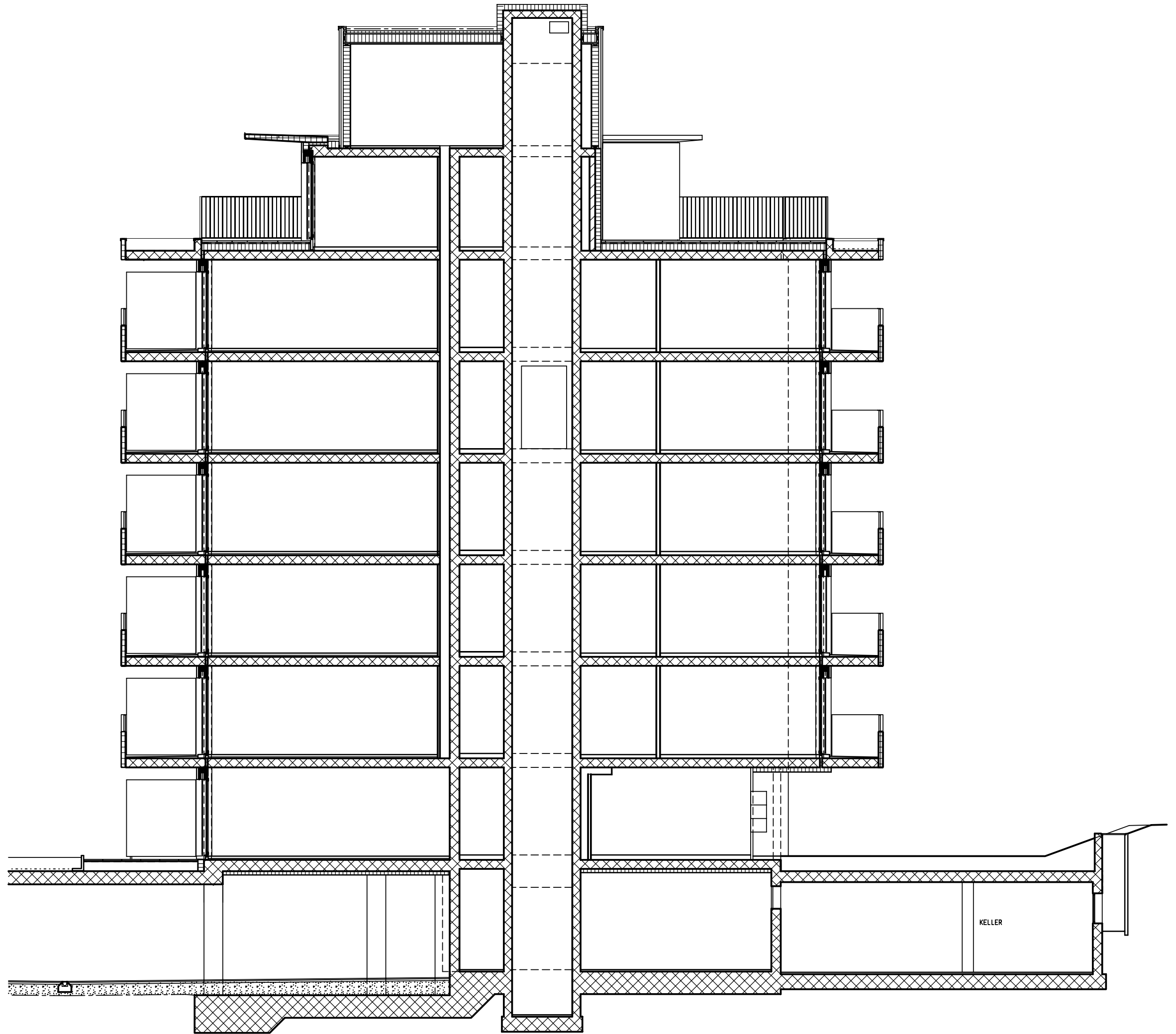
HAUS 1 SCHNITT 1:100
