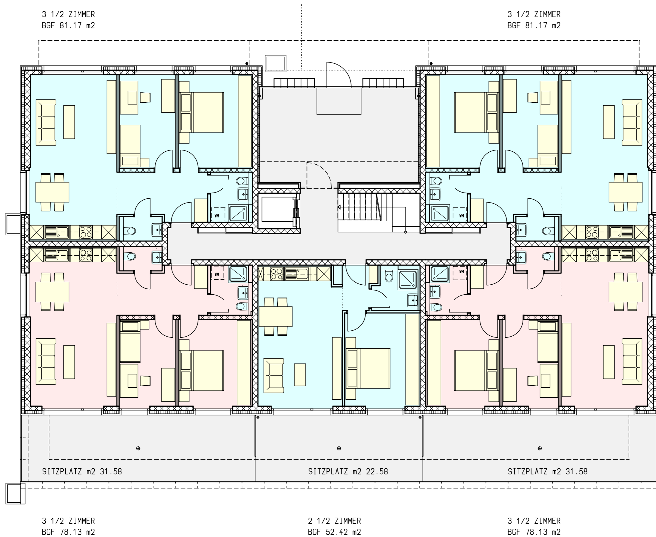
HAUS 1 GARTENGESCHOSS 1:100
